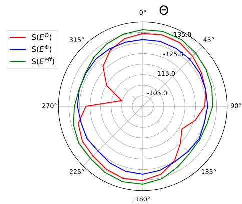
(d) yz-plane
