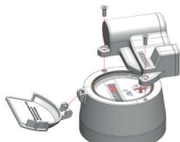
Obr. 5: Montáž EDC-S na měřičím zařízení z mědi/skla (IP68)
