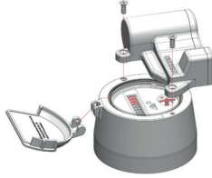
Bild 5: Installation av EDC-S på mätare med koppar-/glas-index (IP68)
