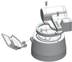
Ill. 4: Montage du modèle EDC-C
