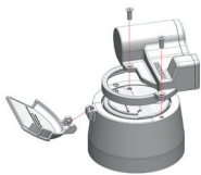
Obr. 4: Montáž EDC-C
