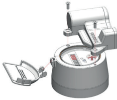
Ill. 5: Montage du modèle EDC-S sur le compteur avec totalisateur verre/métal (IP68)
